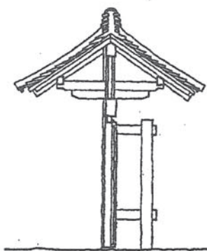
腕木門
