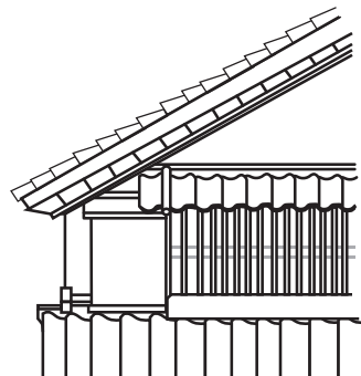
屋根付格子
