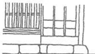
布石敷
