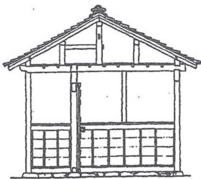
長屋門
