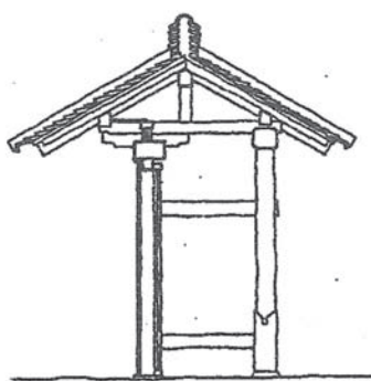
薬医門
